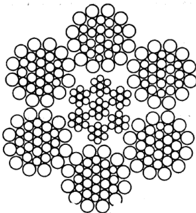
Шестипрядный канат 6 \times 31 + 1 м. с.; 6 \times 31 = 186 проволок с металлическим сердечником конструкции 7 \times 7 = 49 проволок (прядь каната 1 + 6 + 6.6 + 12 ; прядь сердечника 1 + 6 ).
